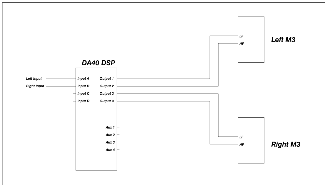
图 4：典型立体声 M2 MkII 系统搭配 DA40 DSP 放大器
