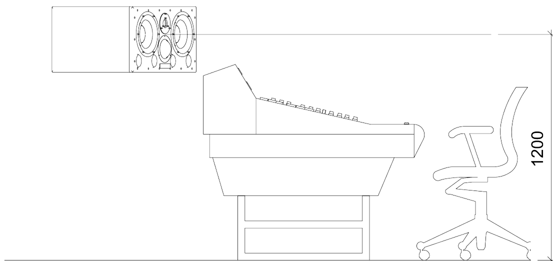
图 5a：典型立体声 M2 MkII 布局 - 侧视图
