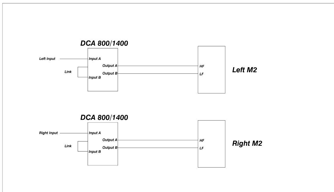
图 3：典型立体声 M2 MkII 系统搭配 DCA 放大器（带滤波器）
