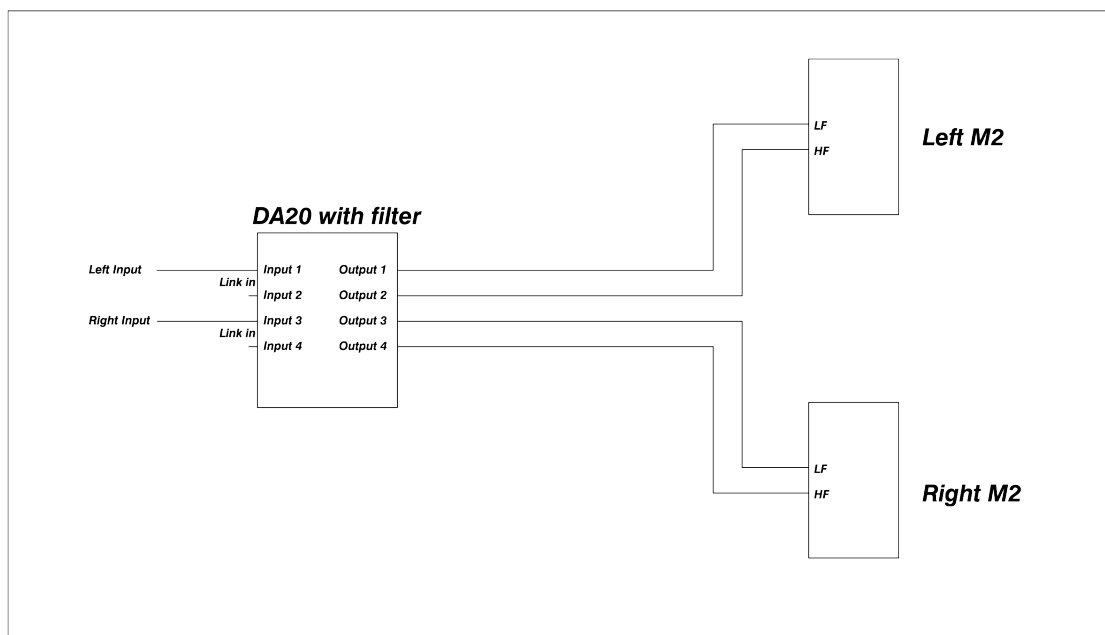
图 2：典型立体声 M2 MkII 系统搭配 DA20 放大器（带滤波器）
