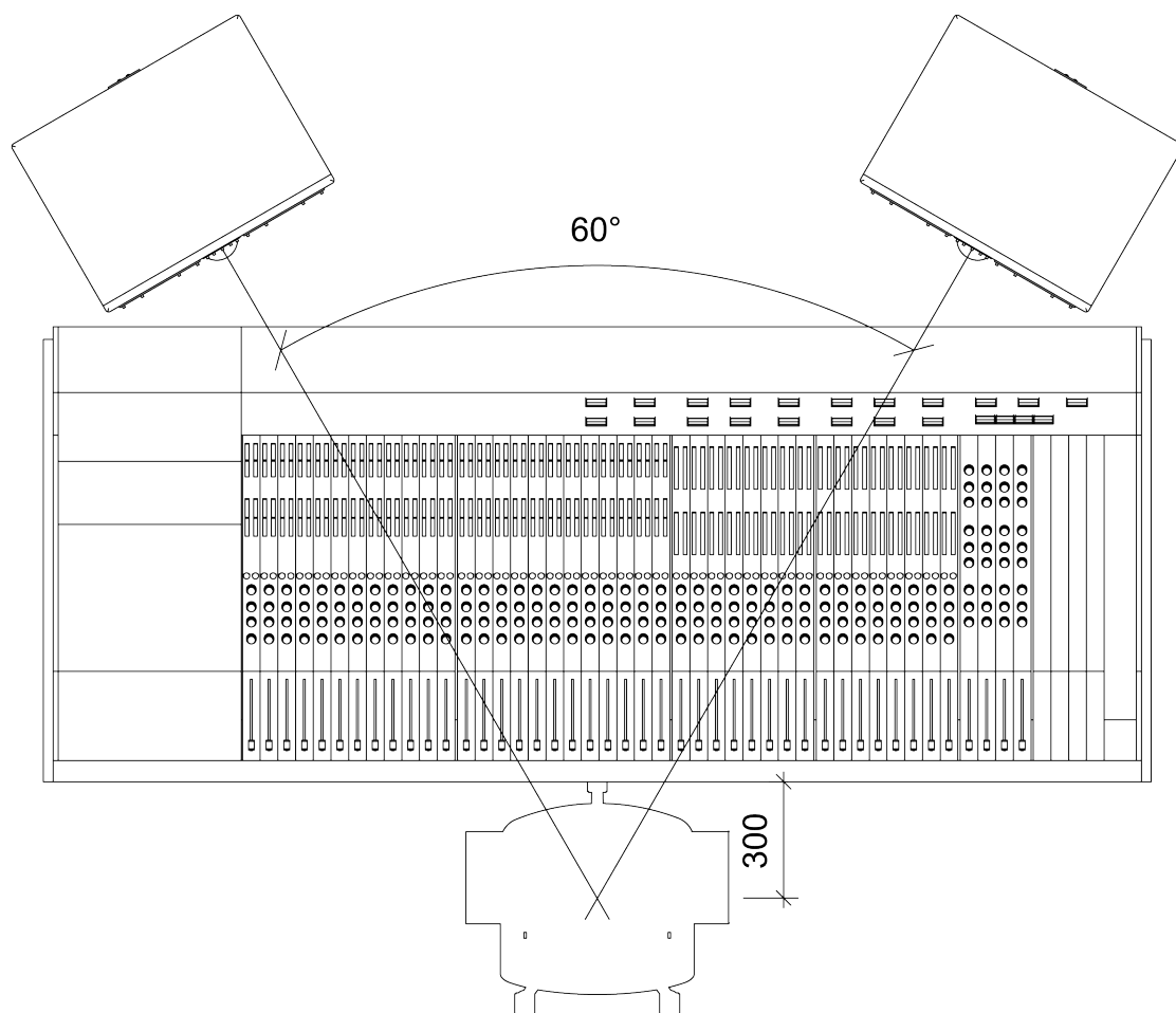
图 5b：典型立体声 M2 MkII 布局 - 俯视图
