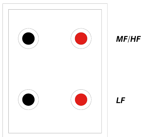
图 1：M2 MkII 连接器面板，红色表示 +ve
