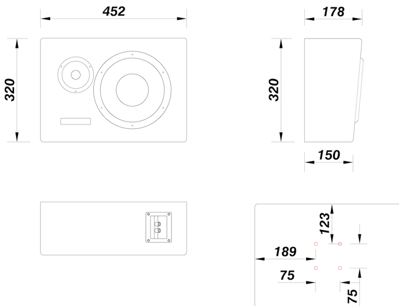
图 3a: MF15c 箱体尺寸及固定点
