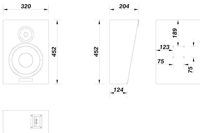
图 3b: MF15c 箱体尺寸及固定点
