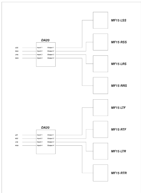
图 2：典型 8 声道环绕声示意图，可能出现在 Dolby Atmos HE 7.1.4 系统中
